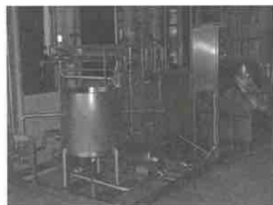
ชุดเครื่องจักรผลิตนมพาสเจอร์ไรส์
